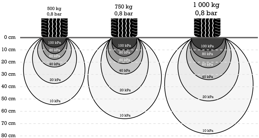
Kuva 4. Rengaskuorman aiheuttama jännitys (paine) maassa.
