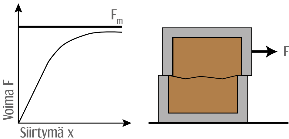
Kuva 1. Maan leikkauslujuus. Kun ylemmää astiaa vedetään, leikkautumiseen tarvittava voima kasvaa ylemmän astian siirtymän pidentyessä. Maa leikkautuu astioiden saumakohdasta.
